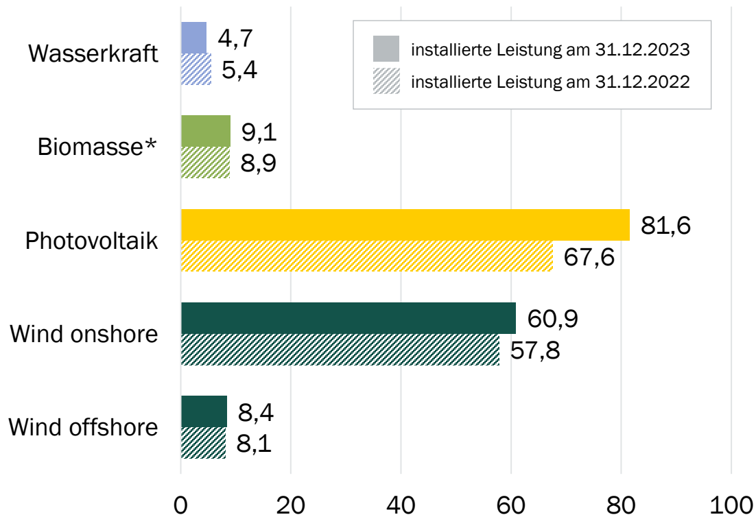
Installierte Leistung erneuerbarer Energien in Deutschland 31.12.2022 und 31.12.2023 [GW]
